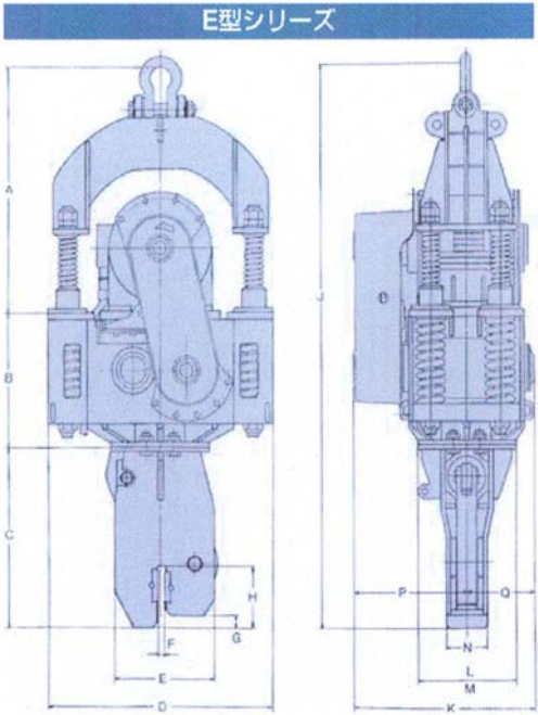
■外形寸法 (単位mm)
